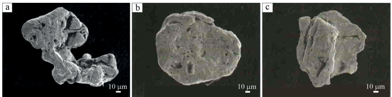
Рис. 4. Морфология золота участка Ойка: окатанная частица сложной формы (а), слабоокатанная и неокатанная частицы пластинчатой формы (b, c). Съемка в режиме вторичных электронов
