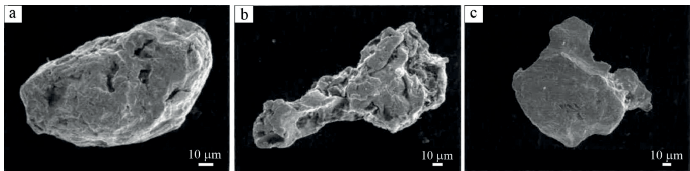
Рис. 5. Морфология золота участка Боровой: окатанные частицы комковидной и сложной удлиненной форм (a, b), неокатанная частица чешуйчатой формы (c). Съемка в режиме вторичных электронов
