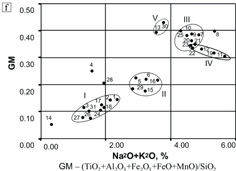
Рис. 1. Некоторые типы пород из артинских последовательностей Косью-Роговской впадины: а–с – скв. Кочмесская-3, гл. 1522.4 м, обр. 9/1; а – спикуловый известняк кремнелый с глинисто-алевро-песчаной примесью (сканированный шлиф), b – деталь (а), шлиф без анализатора; c – с анализатором; d, e – скв. Падимейская-1, гл. 1415.5 м, обр. 4/2; d – тонкие циклиты алевролитов и аргиллитов с градационной слоистостью (сканированный шлиф), e – деталь (d), шлиф без анализатора; f – модульная диаграмма: гидролизатный модуль (GM) – сумма щелочей ( \text{Na}_2\text{O} + \text{K}_2\text{O} ) по [16]
