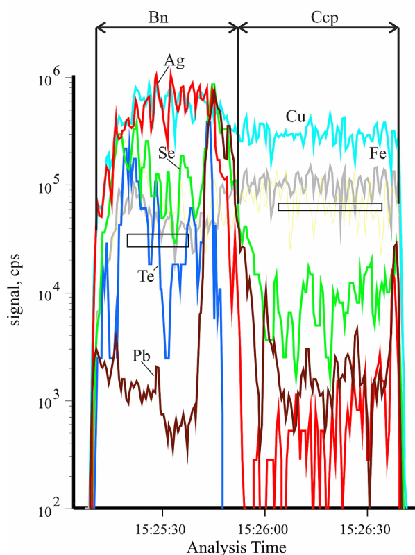
Рис. 11. Распределение элементов-примесей по профилю лазерного микроанализа в сростании «халькопирит-борнит» (ОЯ-12). Примеси концентрируются главным образом в борните и составляют: Se = 6630 ppm, Ag = 3660 ppm, Te = 300 ppm; Pb локализуется в контактовой части минералов. В халькопирите примесей на порядок меньше. Коэффициенты корреляции Ag-Te-Se = 0.7–0.8
