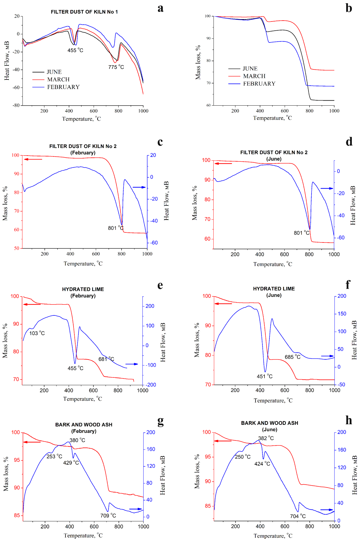
Рис. 3. Кривые нагрева образцов пыли электрофильтров печи № 1 (а, б), печи № 2 (с, д), гашеной извести, полученной из некондиционного оксида кальция (е, ф), кородревесной золы (г, h), отобранных в разное время
