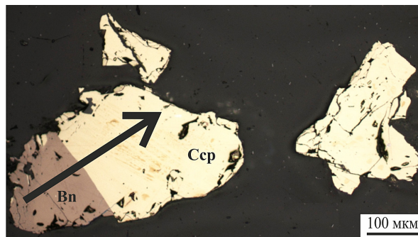
Рис. 11. Распределение элементов-примесей по профилю лазерного микроанализа в сростании «халькопирит-борнит» (ОЯ-12). Примеси концентрируются главным образом в борните и составляют: Se = 6630 ppm, Ag = 3660 ppm, Te = 300 ppm; Pb локализуется в контактовой части минералов. В халькопирите примесей на порядок меньше. Коэффициенты корреляции Ag-Te-Se = 0.7–0.8
