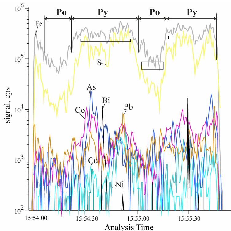
Рис. 10. Распределение элементов-примесей по профилю лазерного микроанализа (линия прожига показана стрелкой, аналогично на рис. 11 и 12) в пирите, «пятнами» замещенном пирротинном (скв.529/169). Элементы-примеси содержатся в повышенных количествах главным образом в пирите: Co = 140–200 ppm, Ni = 100–170 ppm, As = 10–25 ppm, Ag — до 5 ppm, иногда появляются пики Bi, обусловленные, вероятно, микровключениями
