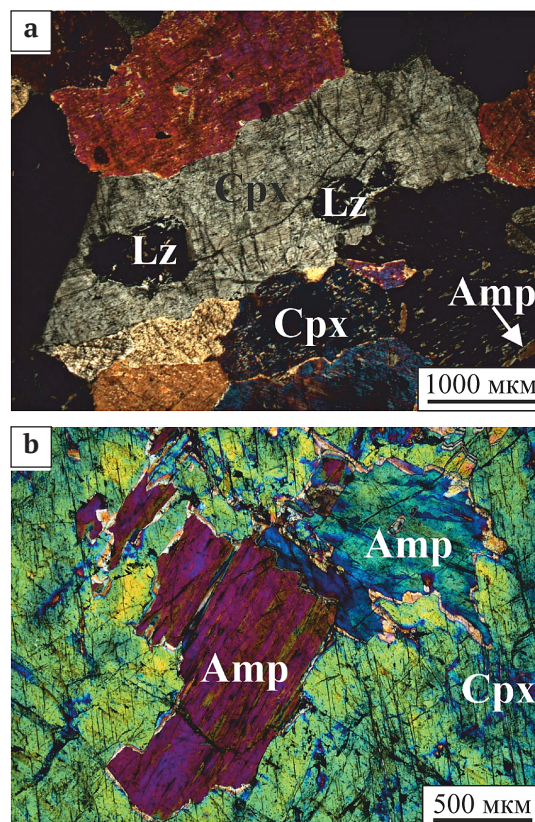
Рис. 4. Характер изменений минерализованных клинопироксенитов и верлитов Озёрного рудопроявления: а — хадакristаллы серпентинизированного и замещенного лизардитом оливина (Lz) в клинопироксене (Cpx), частично замещенном амфиболом (Amp), шлиф ОЯ-9; б — амфиболитизация клинопироксена по массе кристалла, шлиф ОЯ-48-2. Изображения в проходящем свете, николи скрещены
