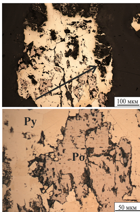
Рис. 10. Распределение элементов-примесей по профилю лазерного микроанализа (линия прожига показана стрелкой, аналогично на рис. 11 и 12) в пирите, «пятнами» замещенном пирротинном (скв.529/169). Элементы-примеси содержатся в повышенных количествах главным образом в пирите: Co = 140–200 ppm, Ni = 100–170 ppm, As = 10–25 ppm, Ag — до 5 ppm, иногда появляются пики Bi, обусловленные, вероятно, микровключениями
