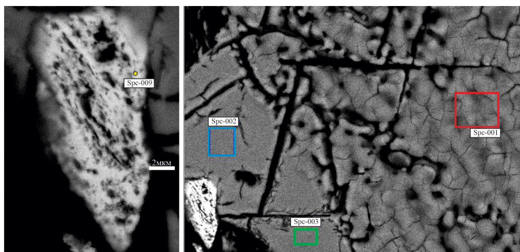
Рис. 9. Включение теллурида палладия (светлое включение состава C_{Pd} \approx C_{Te} , вероятнее всего котульскит) в халькопирите, слева — увеличенный фрагмент с изображением включения (ОЯ-28-2)
