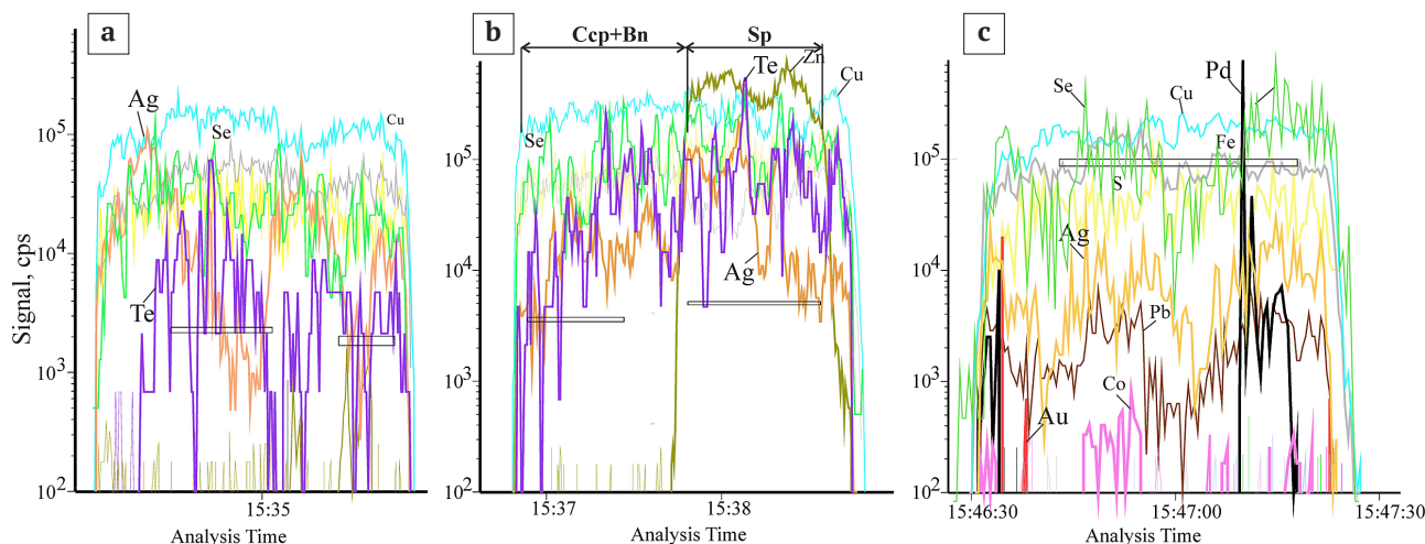
Рис. 12. Распределение элементов-примесей по профилю лазерного микроанализа в минералах продуктивной борнит-халькопиритовой ассоциации (ОЯ-28-1):
