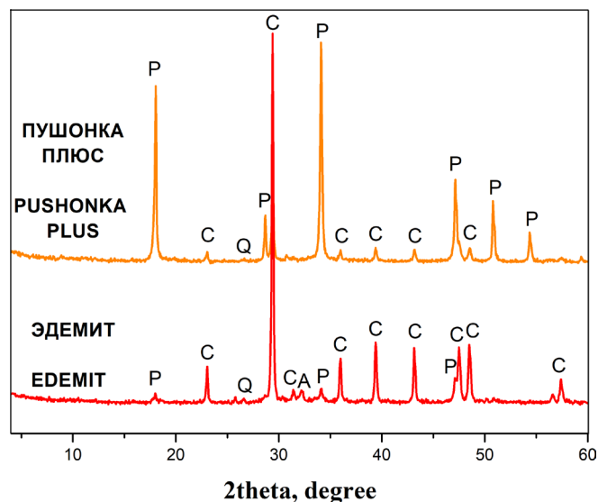
Рис. 4. Дифрактограммы агрохимикатов «Эдемит» и «Пушонка плюс». P — портландит, C — кальцит, A — апатит, Q — кварц
