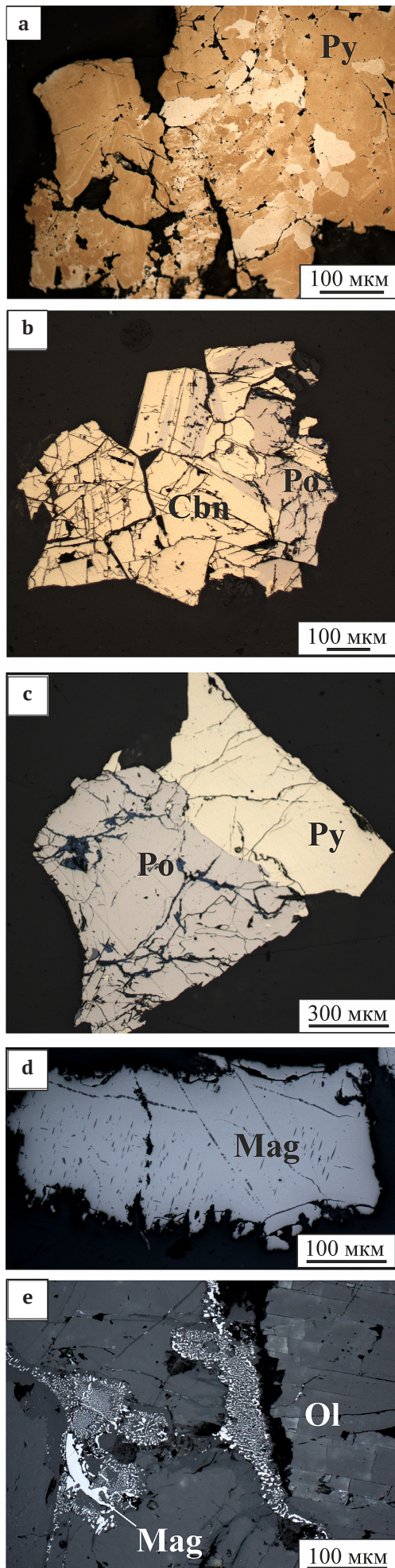
Рис. 7. Взаимоотношения минералов пирротин-халькопирит-кубанитовой ассоциации:
