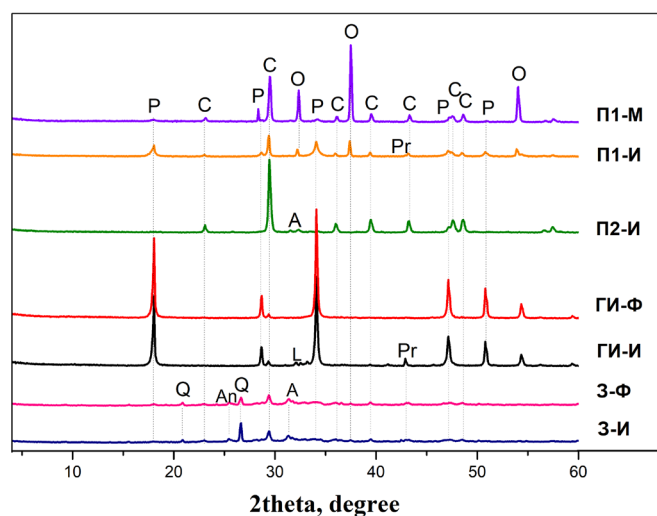
Рис. 2. Дифрактограммы вторичного минерального сырья: P — портландит, C — кальцит, O — оксид кальция, A — апатит, Pr — периклаз, Q — кварц, An — ангидрит
