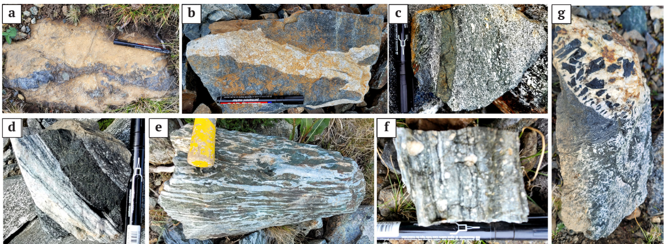
Рис. 3. Взаимоотношения магматических образований и их изменения: а — пересечение оливинитов клинопироксенитами; б–д — дайкоподобные образования разного состава в измененных габброидах; е — амфиболизированные габброиды с директивной текстурой; ф — аполейкоплагиогранитовые бластомилониты, г — контакт тулитовых габбро с амфиболизированными габброидами
