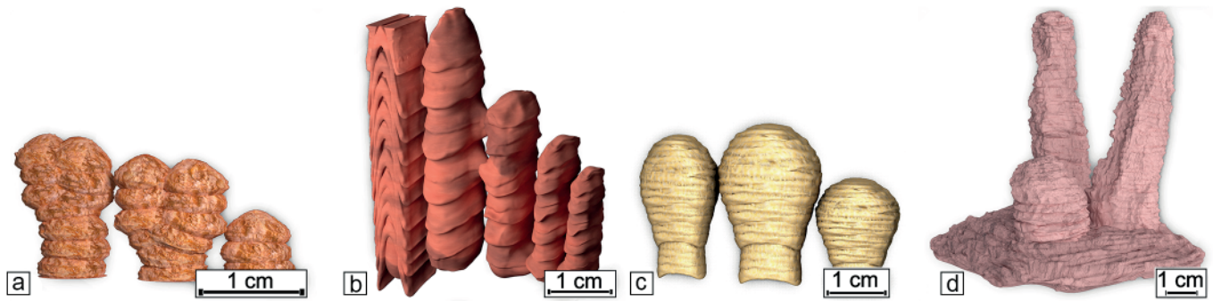
Рис. 10. 3D-модели палеопротерозойских строматолитов, созданные с помощью программы Blender: а — Djulmekella ; б — Segosia ; в — Omachtenia ; г — Severinsaaria gen. nov.
