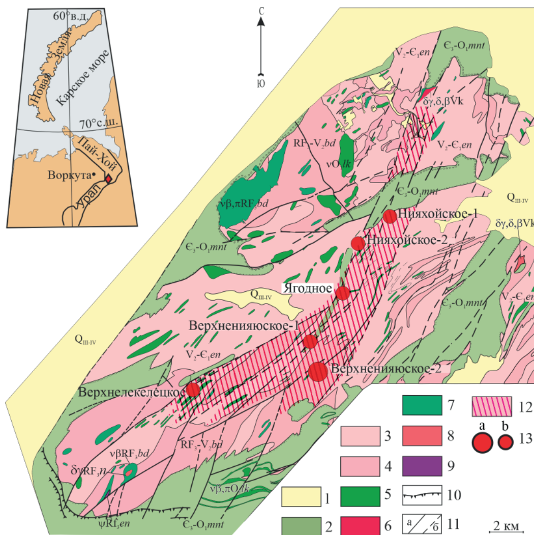
Рис. 1. Геологическое строение и золоторудные проявления Манитаньрдского района (Государственная..., 2013 с дополнениями): 1 — четвертичные отложения; 2 — манитаньрдская серия нерасчлененная (верхний кембрий — нижний ордовик); 3 — энганепэйская* свита (верхний венд — нижний кембрий); 4 — бедамельская серия нерасчлененная (верхний рифей — венд). Интрузивные образования: 5 — леквозжский комплекс: оливиновые габбро и долериты, пикродолериты; 6 — кызыгейский комплекс: диориты, гранодиориты, плагиограниты; 7 — нижнебедамельский комплекс: габбро, габбро-долериты; 8 — нияюский комплекс: диориты, гранодиориты, плагиограниты; 9 — энганепэйский комплекс: серпентиниты апоперидотитовые, апиноксенитовые; 10 — тектонические покровы; 11 — разрывные нарушения: а — достоверные, b — предполагаемые; 12 — Нияюская рудная зона; 13 — золоторудные месторождения (а) и проявления (b)
