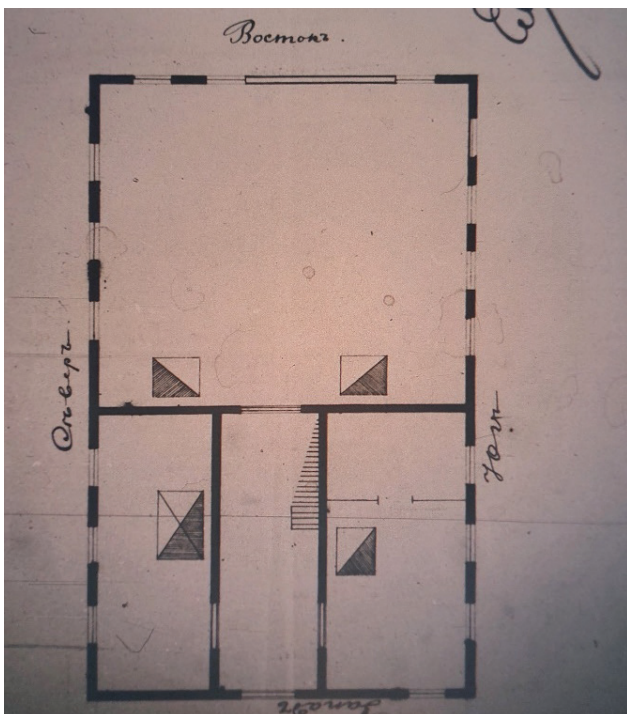
Рисунок 2. План церковно-приходской школы при Спасо-Преображенской церкви в селе Малая Пинега. Pic. 2. Plan of the parish school at the Church of the Transfiguration of the Savior in the village of Malaya Pinega.
